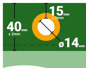
Bande polyéthylène
